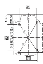
取付寸法図
