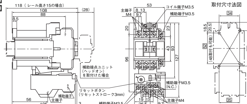
取付穴寸法図
