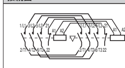
接続図
