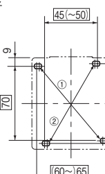
取付寸法図
