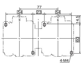
取付穴寸法図
