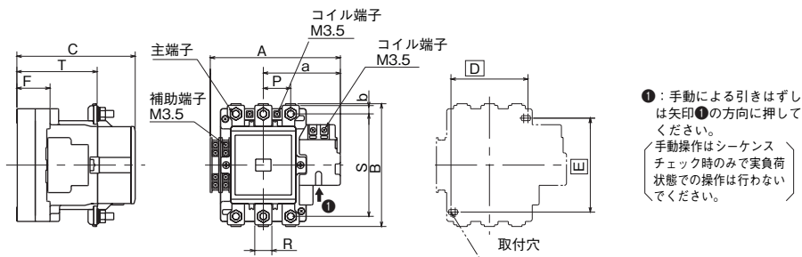
SC-N1/VS, N2/VS形の取付の場合
