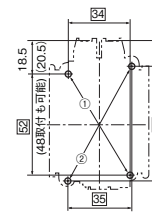
取付寸法図
