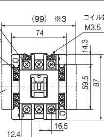
取付寸法図
