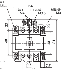
取付寸法図
