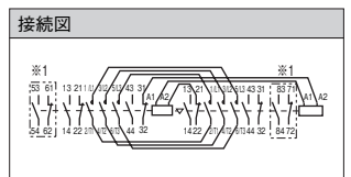
※1 補助接点3a3b×2の場合
