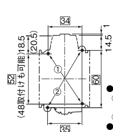
取付寸法図
