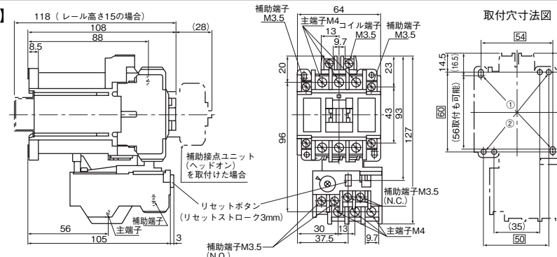
取付穴寸法図
