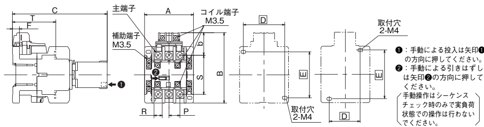
SC-N1/VS, N2/VS形の取付の場合
