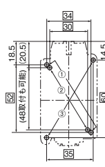
取付寸法図
