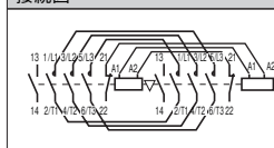
接続図
