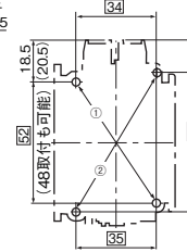
取付穴寸法図
