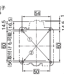
取付寸法図
