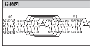
※1 補助接点4a4b×2の場合
