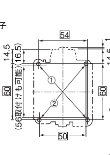
取付寸法図
