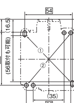
取付寸法図
