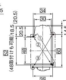
取付寸法図
